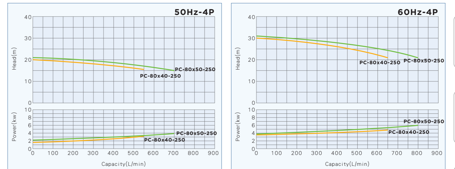
PC-80x40-250 / 80x50-250
