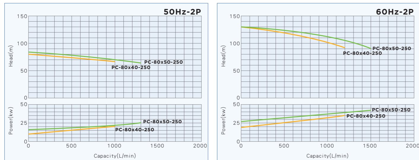
PC-80x40-250 / 80x50-250
